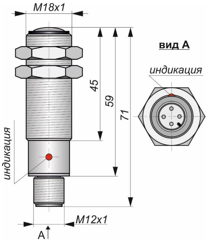
Габаритный чертеж
