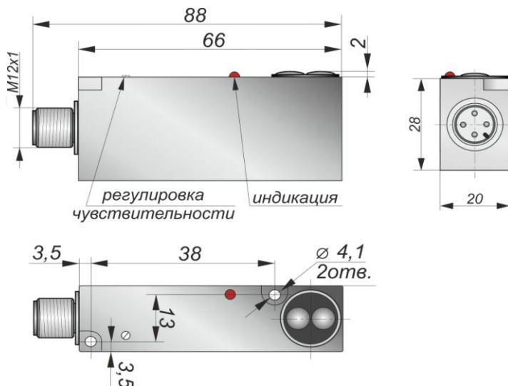
Габаритный чертеж
