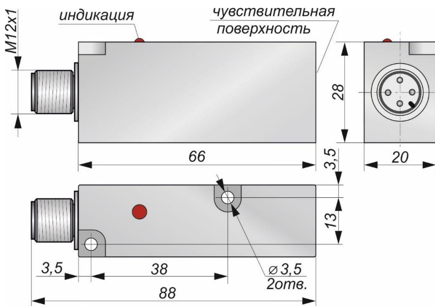
Габаритный чертеж
