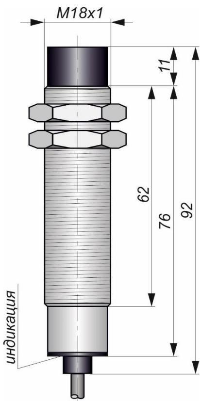
Габаритный чертеж
