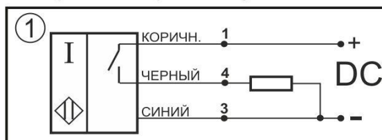
Схема подключения
