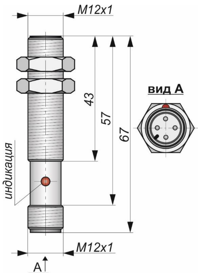
Габаритный чертеж
